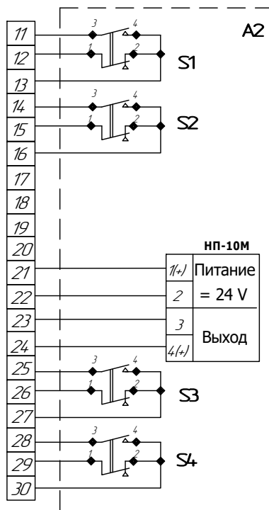
Рисунок Б.2 – Схема механизма с датчиком БСП-2 остальное см рис Б.1
