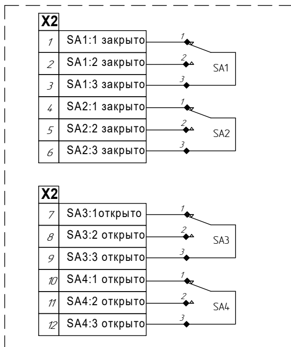
Рисунок Б.1 Схема блока БСПМ-10АК
