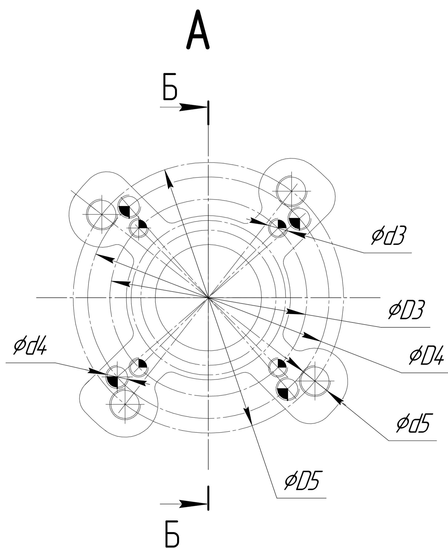
Рисунок А.4 – Общий вид, габаритные и присоединительные размеры механизма МЭОФ-ИСТ4 группы 500 с внутренним присоединением по ISO ГОСТ Р 55510-2013
