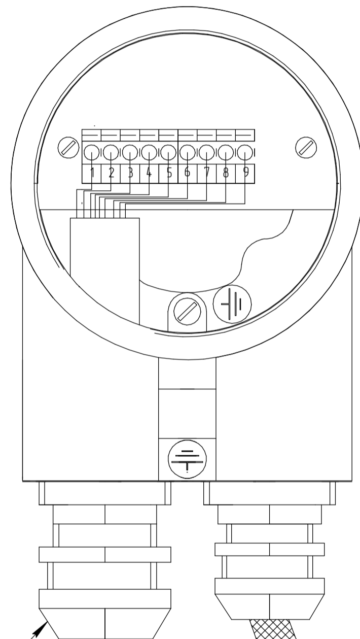
Датчик БЦА-2-ИСТ4
