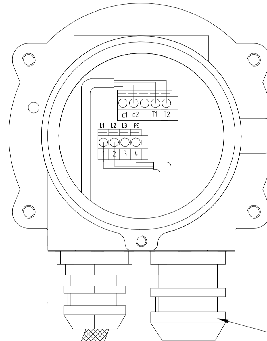
Двигатель ДСР-118-ИСТ4, ДСР-142-ИСТ4
