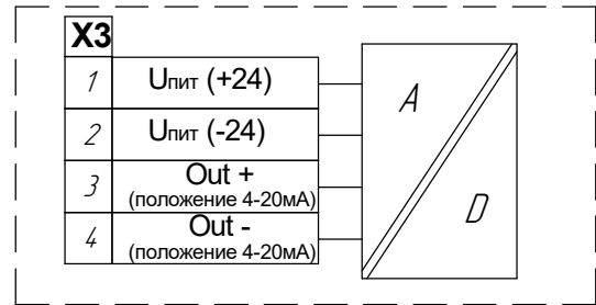
Рисунок Б.2 – Схема механизма с блоком БСПТ-10АК Остальное см. рис. Б.1
