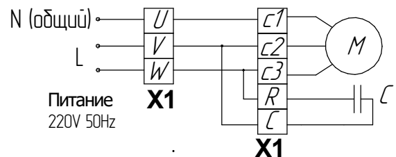
Рисунок Б.5 – Схема механизма однофазного исполнения Остальное см. рис. Б.1, Б.2, Б.3
