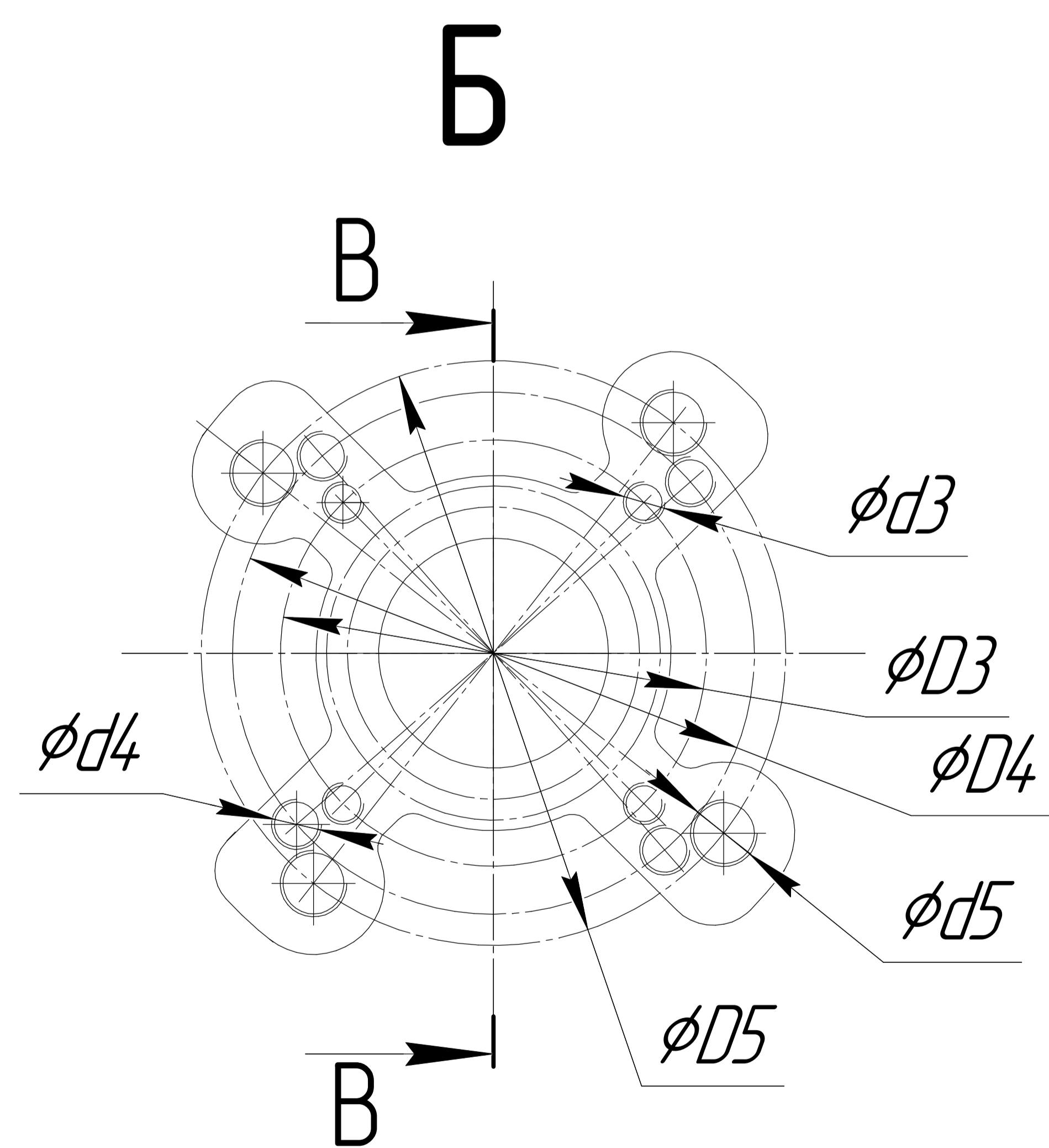
Рисунок А.6 – Механизм М30Ф группы 500-92 с внутренним присоединением по ISO ГОСТ Р 3427-20137 Остальное см. рис. А.5
