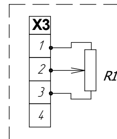
Рисунок Б.3 – Схема механизма с блоком БСПР-10АК Остальное см. рис. Б.1
