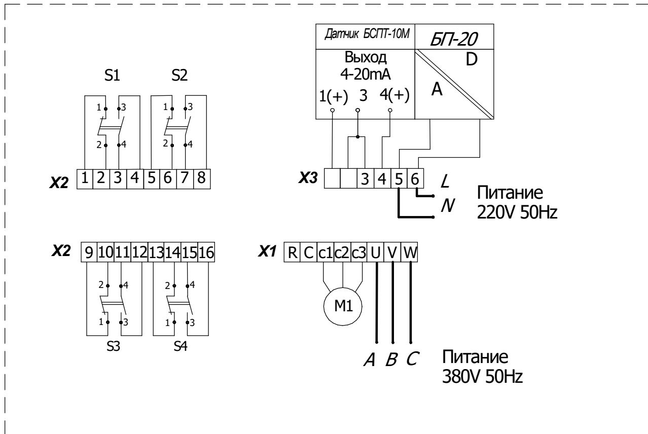
Рисунок Б.5 - Схема механизма МЭО(Ф)-630-КБ трехфазного исполнения с блоком БСПТ-10М со встроенным БП-20
