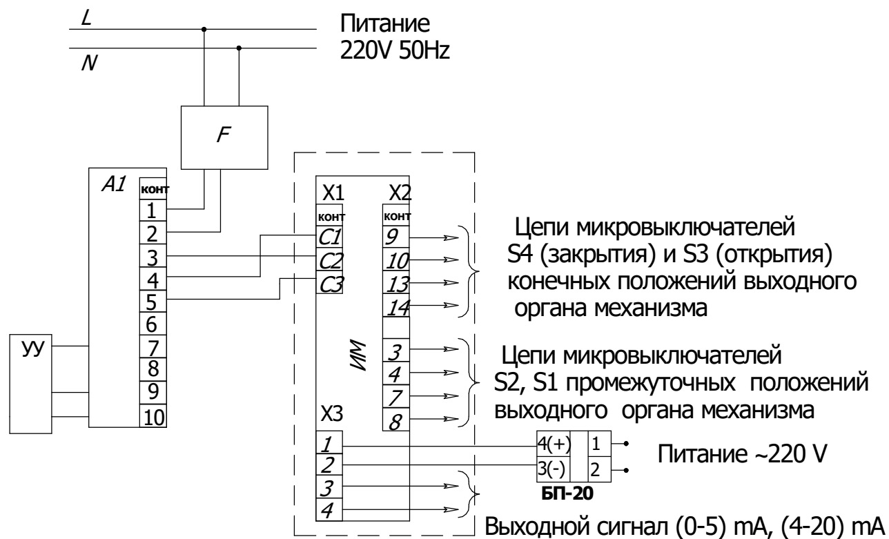
Рисунок В.2- Схема подключения механизма к сети 220V с блоком БСПТ-10М при бесконтактном управлении
