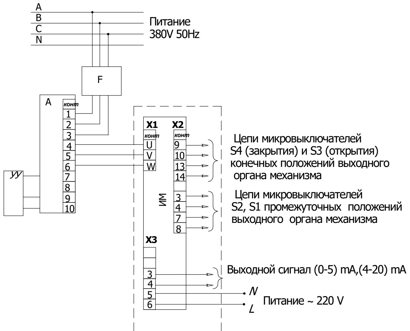
Рисунок В.3 - Схема подключения механизма МЭО(Ф)-630-КБ к сети 380V с датчиком БСРТ-10М на клеммном блоке при бесконтактном управлении
