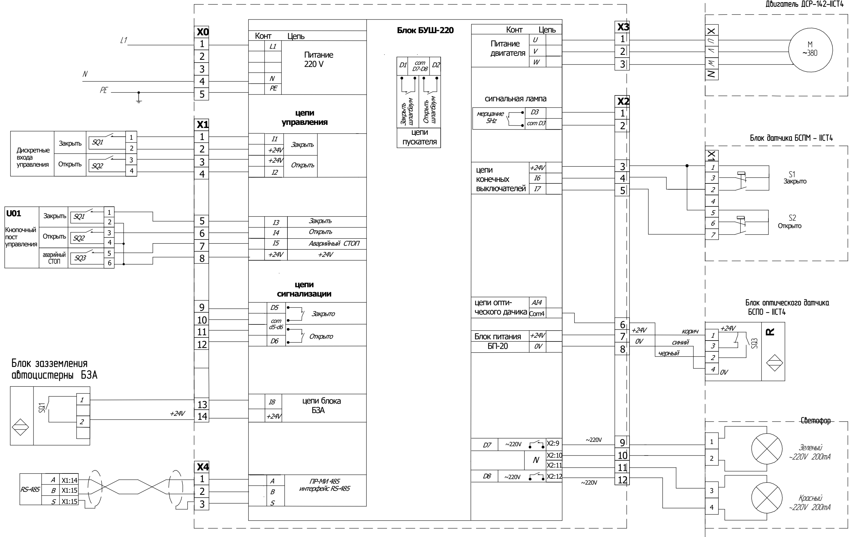
Рисунок В.1 – Схема подключения шлагбаума АШК-ІВТ4 к блоку БУШ-220 с датчиком препятствия и с блоком БЗА
