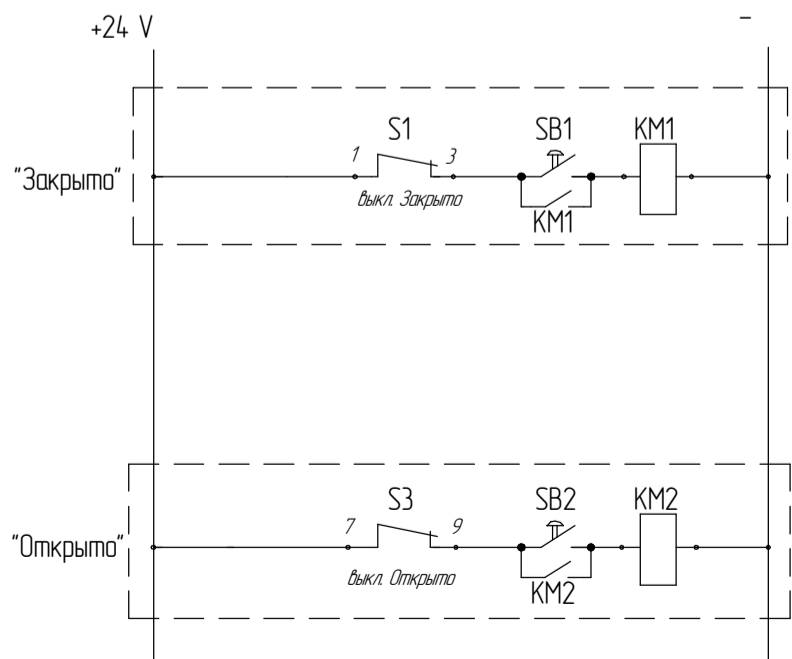
Рисунок В.3 - Схема управления механизма с блоком БСПТ-10АК
