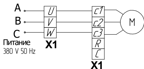
Рисунок Б.4- Схема механизма трехфазного исполнения Остальное смотреть рисунок Б.1, Б.2, Б.3
