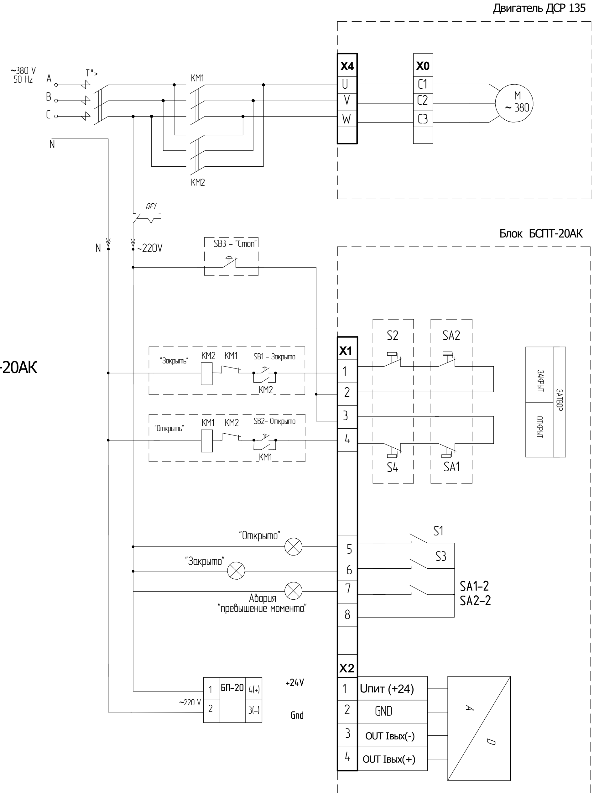
Рисунок В.1 - Схема проверки трехфазного механизма с блоком БСПТ-20АК
