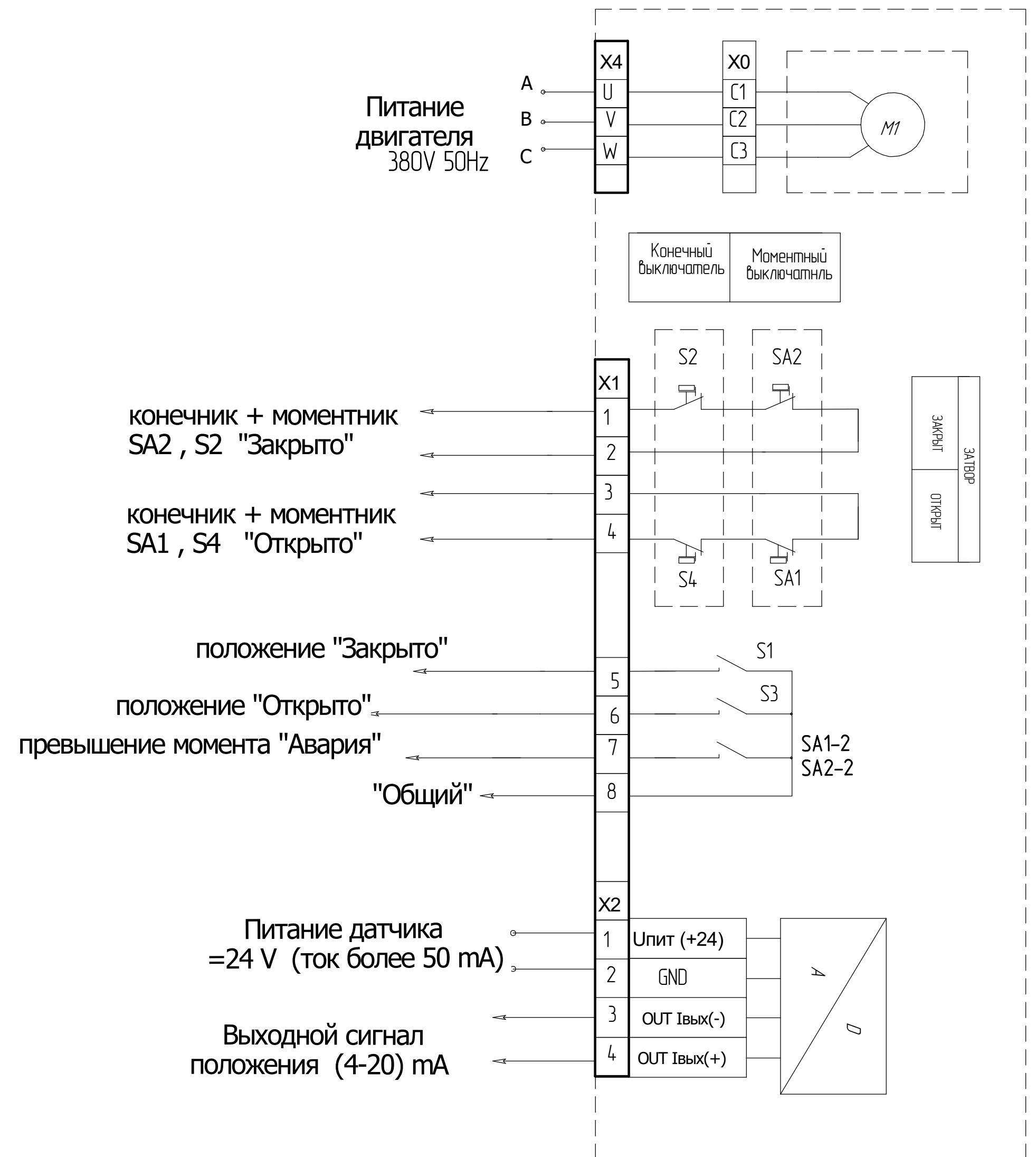
Рисунок Б.1 – Схема трехфазного механизма с блоком БСПТ-20АК
