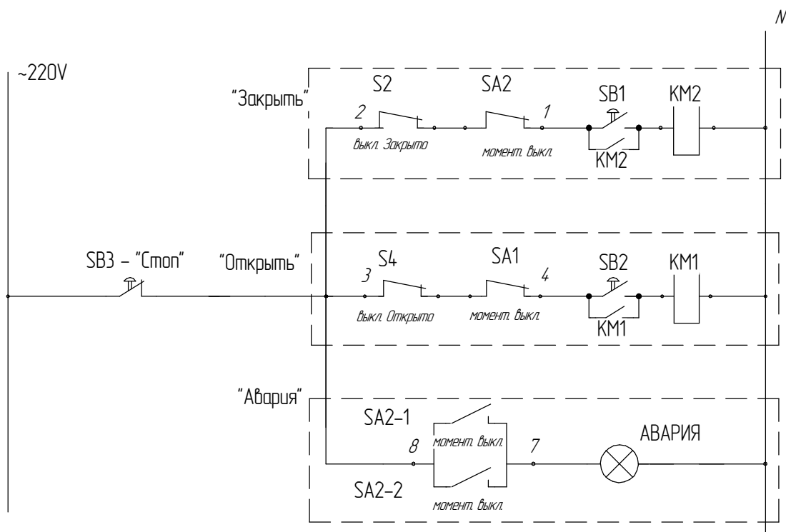
Рисунок В.3 - Схема управления механизма с блоком БСПТ-20АК
