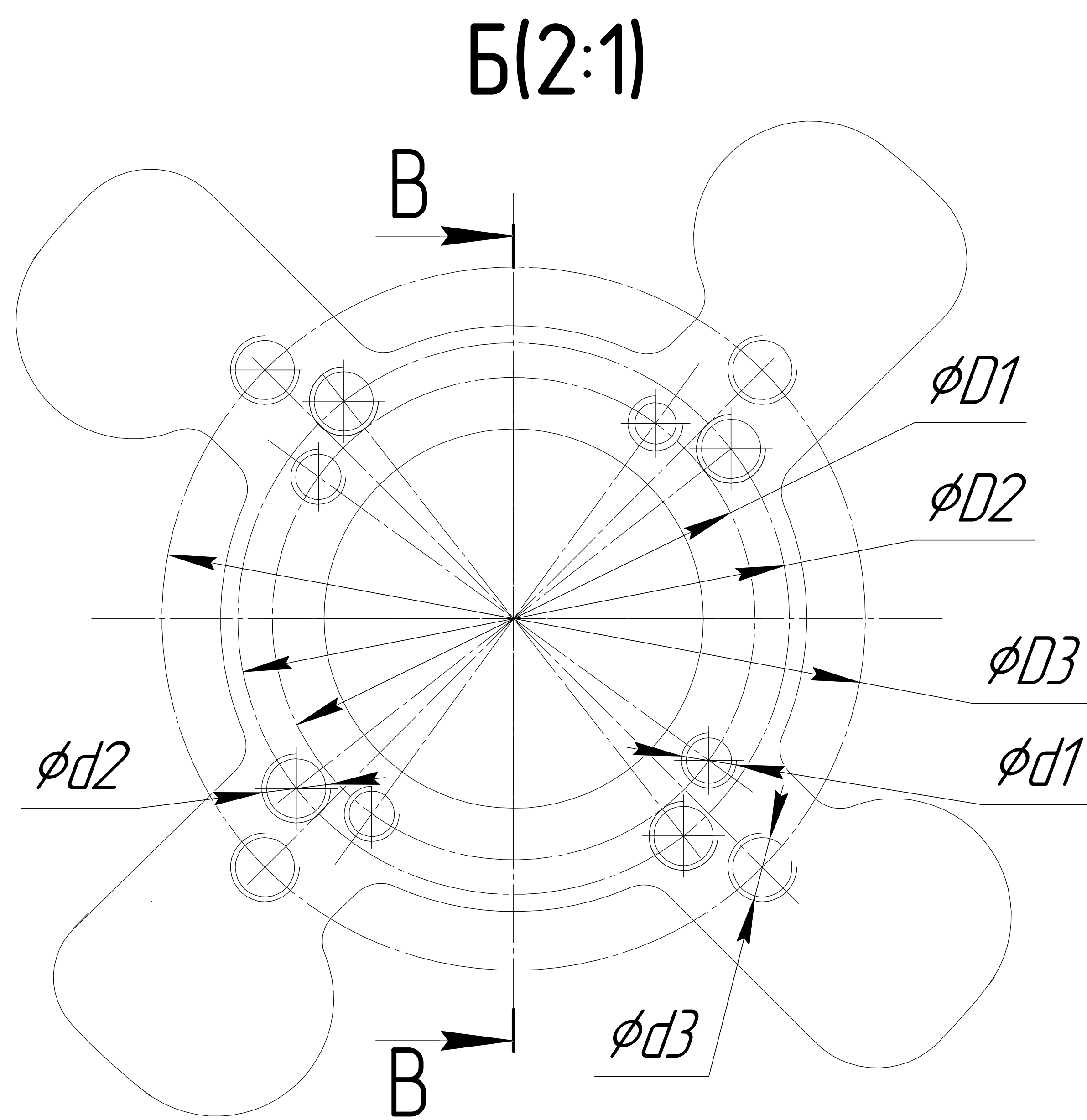
Рисунок А.4 – Механизм МЗОФ группы 250 с внутренним присоединением по ISO ГОСТ Р 34287-2017
