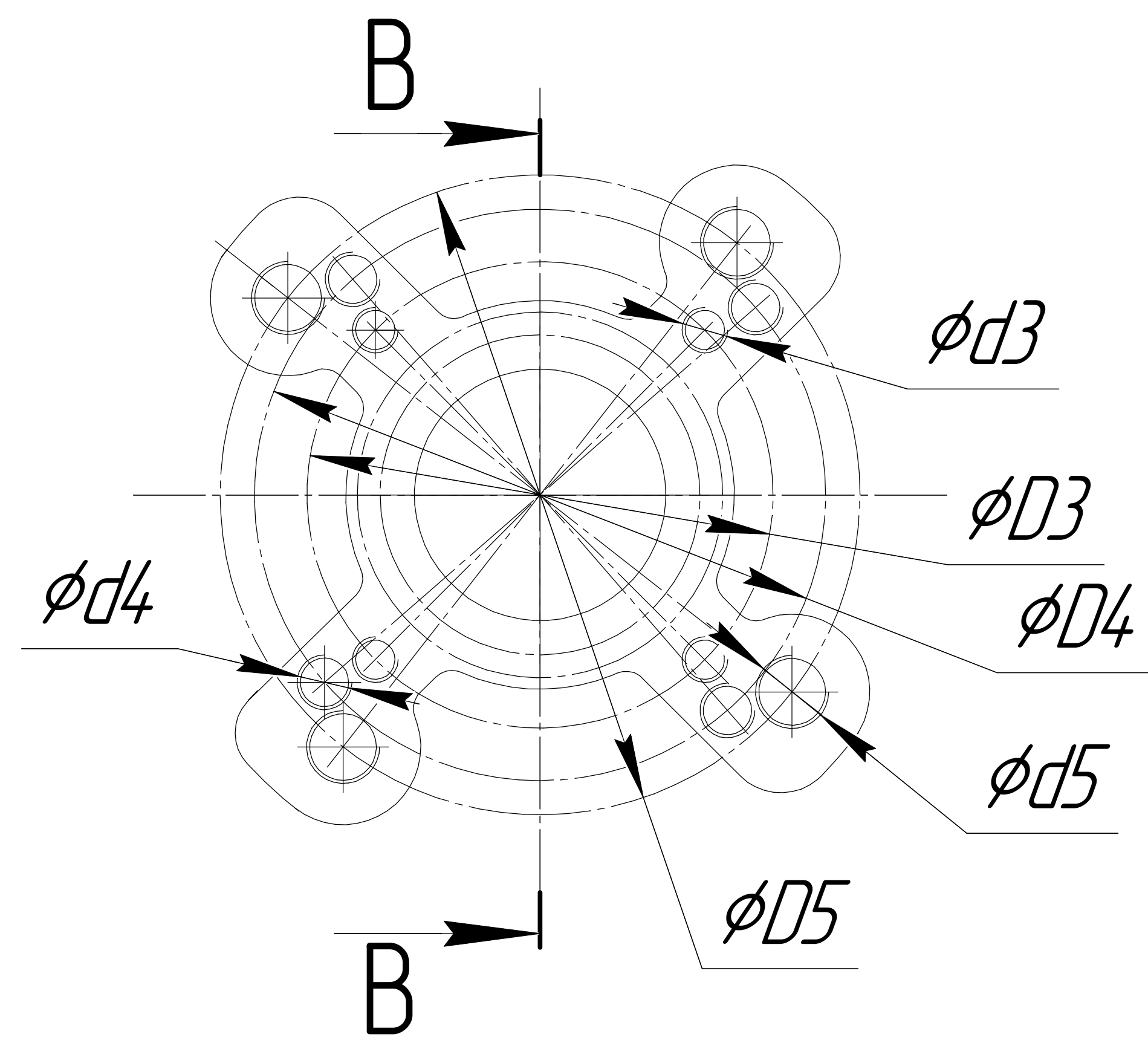
Рисунок А.5 – Механизм МЭОФ группы 500 с внутренним присоединением по ISO ГОСТ Р 34287-2017 Остальное см. рисунок А.4
