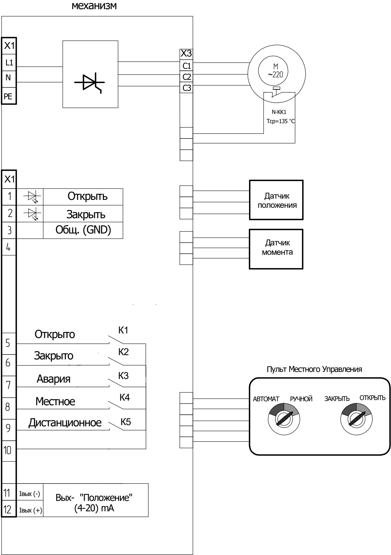
Рисунок В.2 – Схема подключения механизма МЭОФ с блоком ЕД 220
