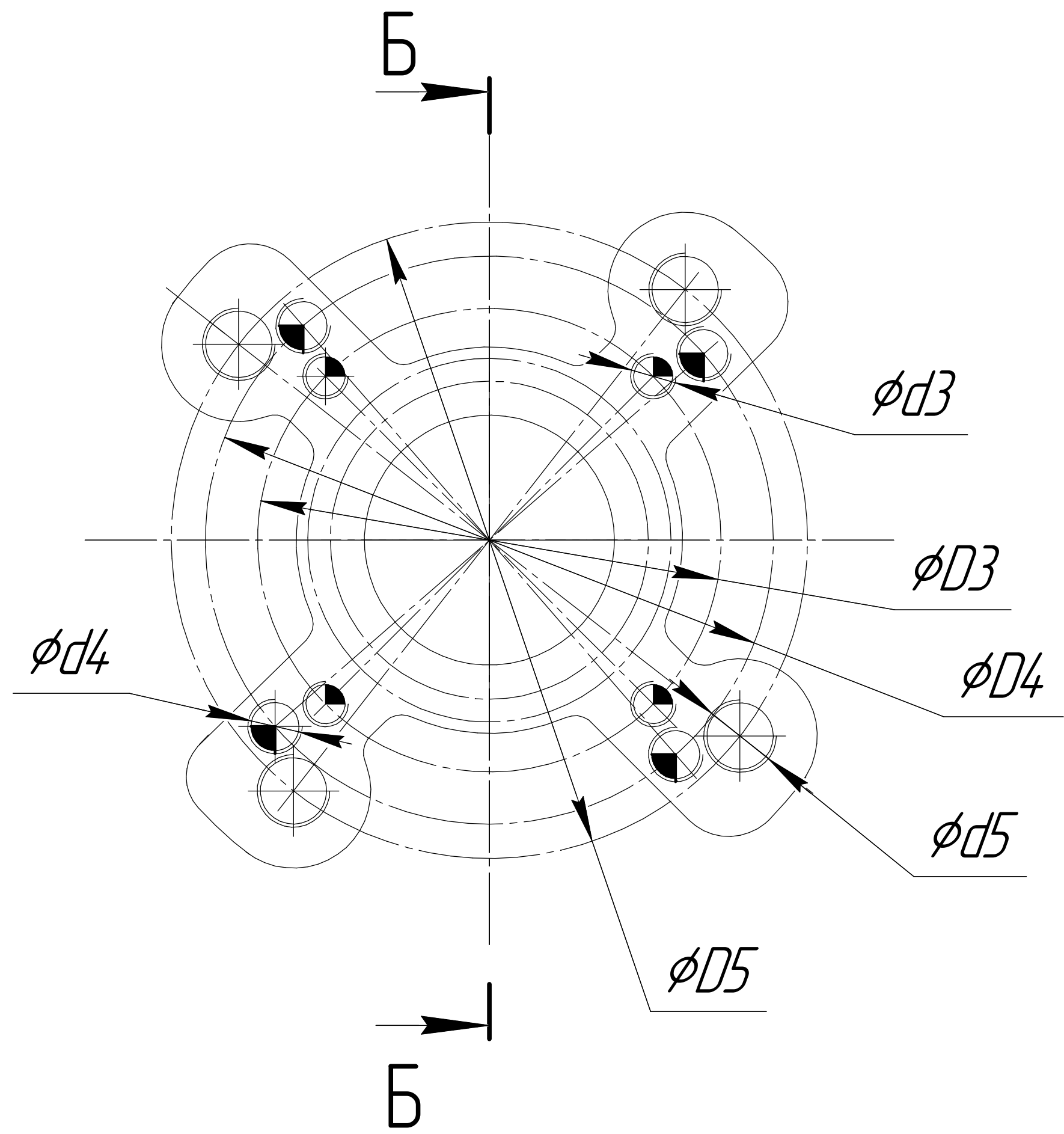
Рисунок А.9 – Общий вид, габаритные и присоединительные размеры механизма МЭОФ– ИСТ4 группы 500 с внутренним присоединением по ISO ГОСТ Р 34287-201, остальное см. рисунок А.8
