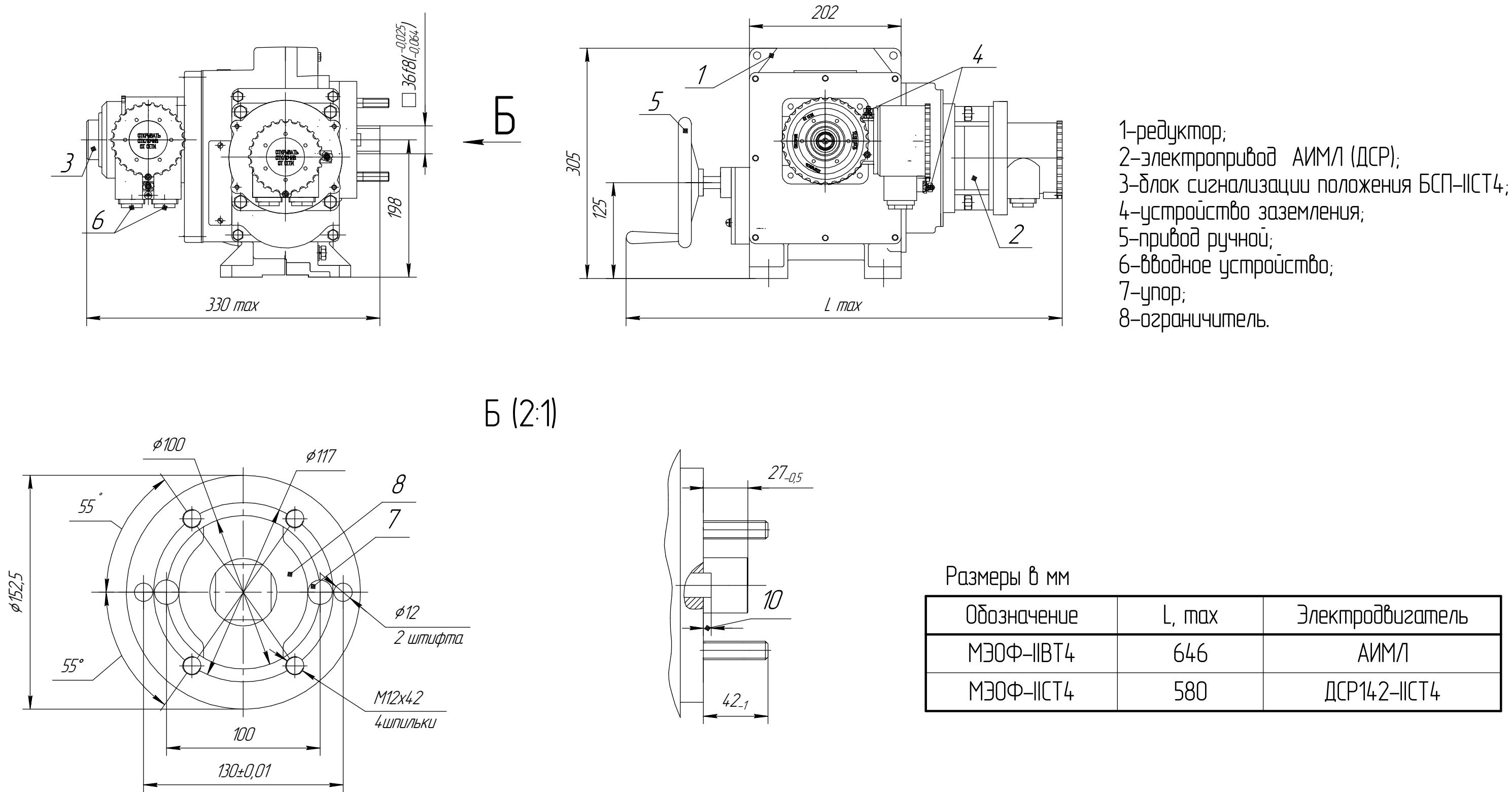
Рисунок А.8 – Общий вид, габаритные и присоединительные размеры механизмов МЭОФ-ИСТ4; МЭОФ-ИВТ4 группы 500 с наружным квадратом выходного вала.
